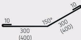
Nr. 182 Skotrenna 300 x 300 Nr. 183 Skotrenna 400 x 400
