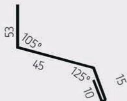
Nr. 660 Dropalisti
