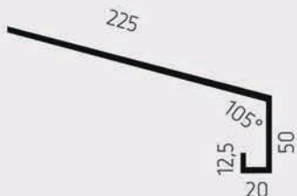
Nr. 651 Vatnsbretti
